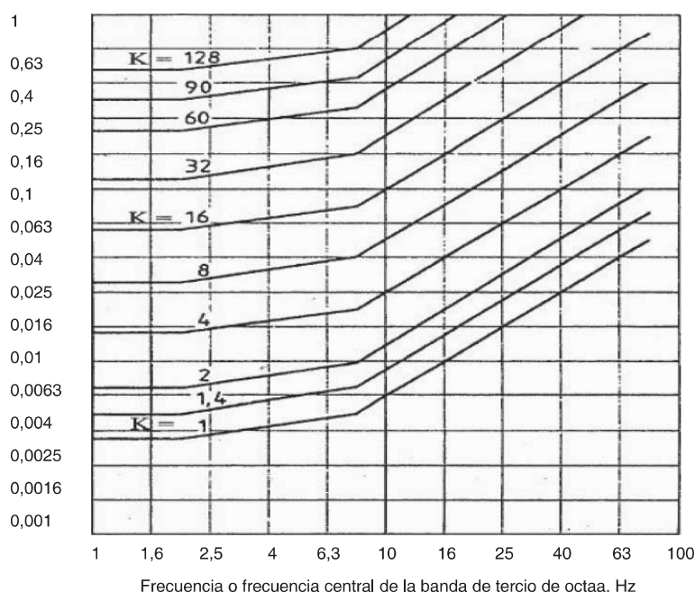
GRÁFICO FACTOR K
